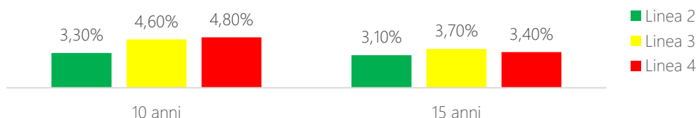
Rendimenti medi annui composti (dati al 31/03/2020)
